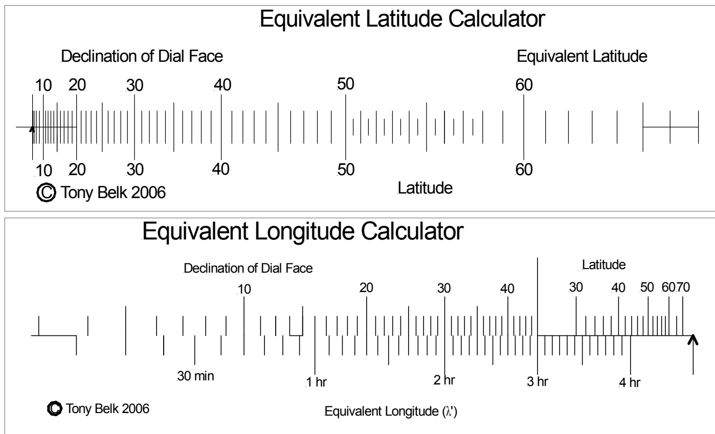
Fig. 1 (top). Equivalent latitude calculator. Fig. 2 (bottom). Equivalent longitude calculator.
